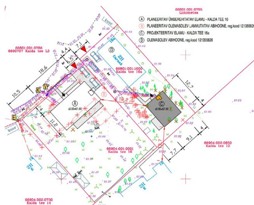
Kalda tee 16a asendiplaani väljavõte (autor Taavi Tuisk, Mereno Ehitus OÜ).
