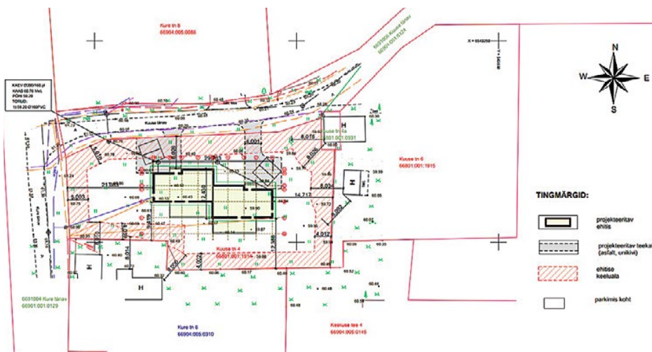
Kuuse tn 4 kavandatava paariselamu asendiskeem (autor arhitekt Jelena Truusa).
