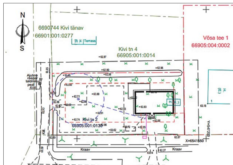
Kivi tn 2 kavandatav asendiplaan (Jaagu Kinnisvara OÜ töö).
