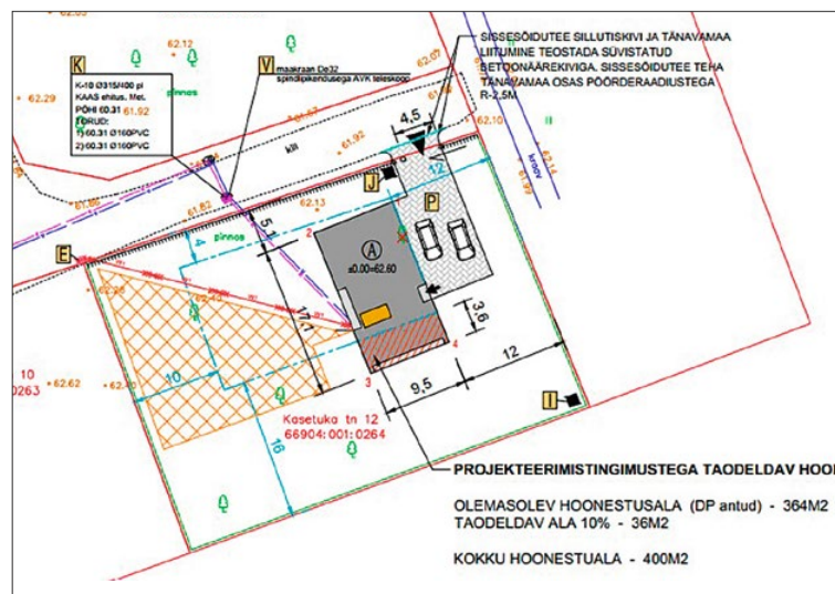
Kasetuka tn 12 kavandatav asendiplaan (Mereno Ehitus OÜ töö).
